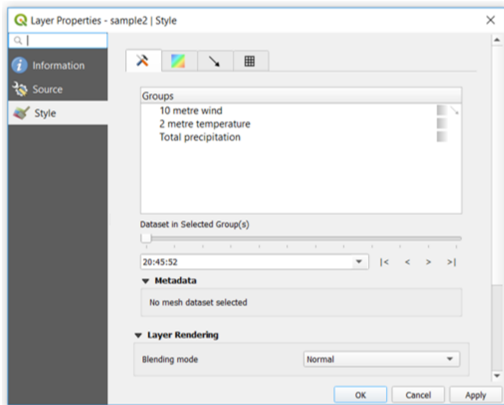
Рис. 15.6: Mesh Layer Style
