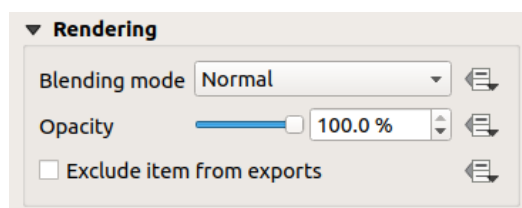
Рис. 16.13: Rendering mode
