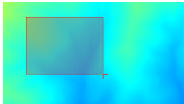
Рис. 21.13: Extent Drag
