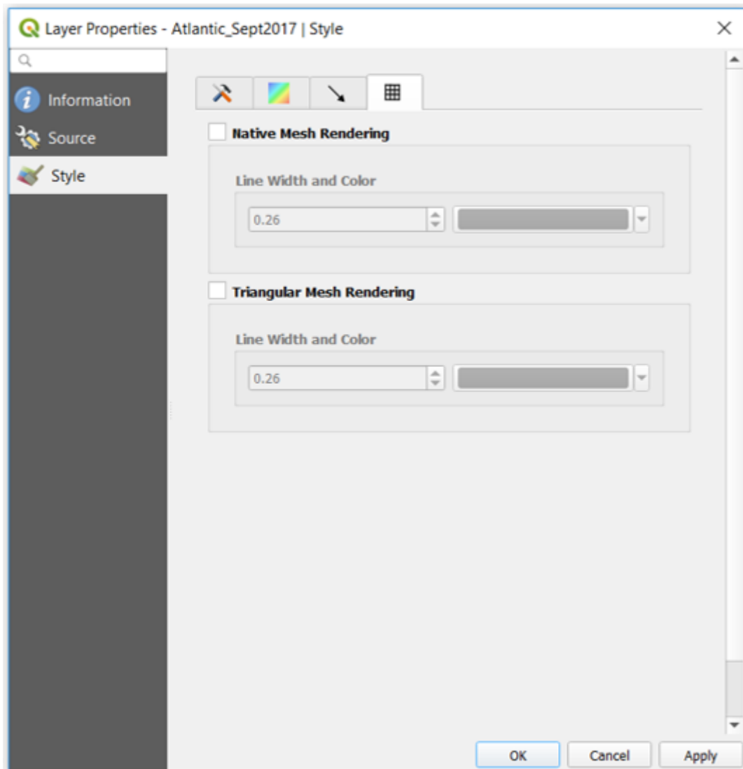
Рис. 15.10: Mesh Rendering
