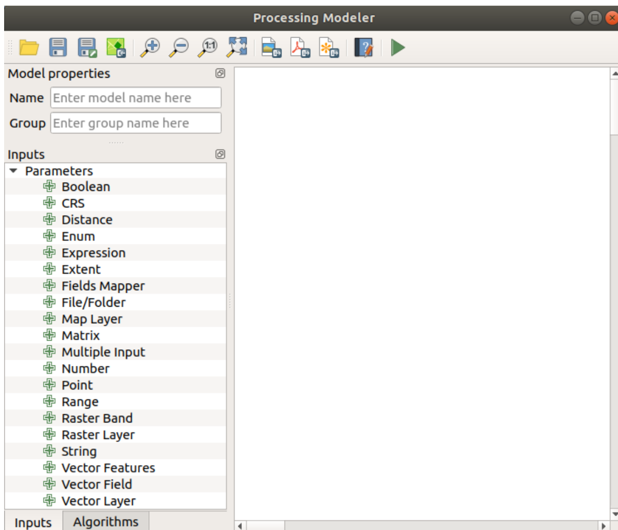
Рис. 21.18: Modeler
