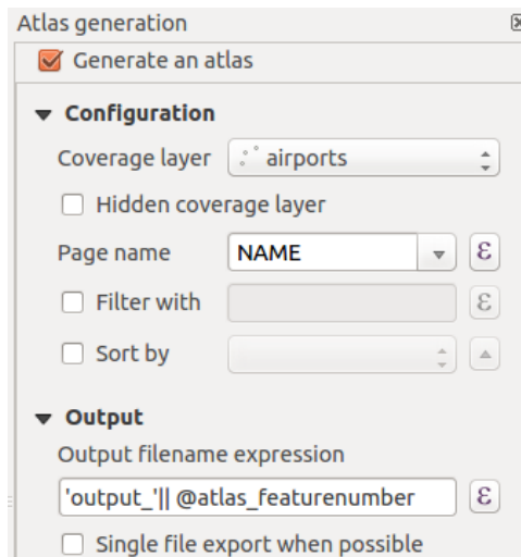
Рис. 16.57: Atlas Panel
