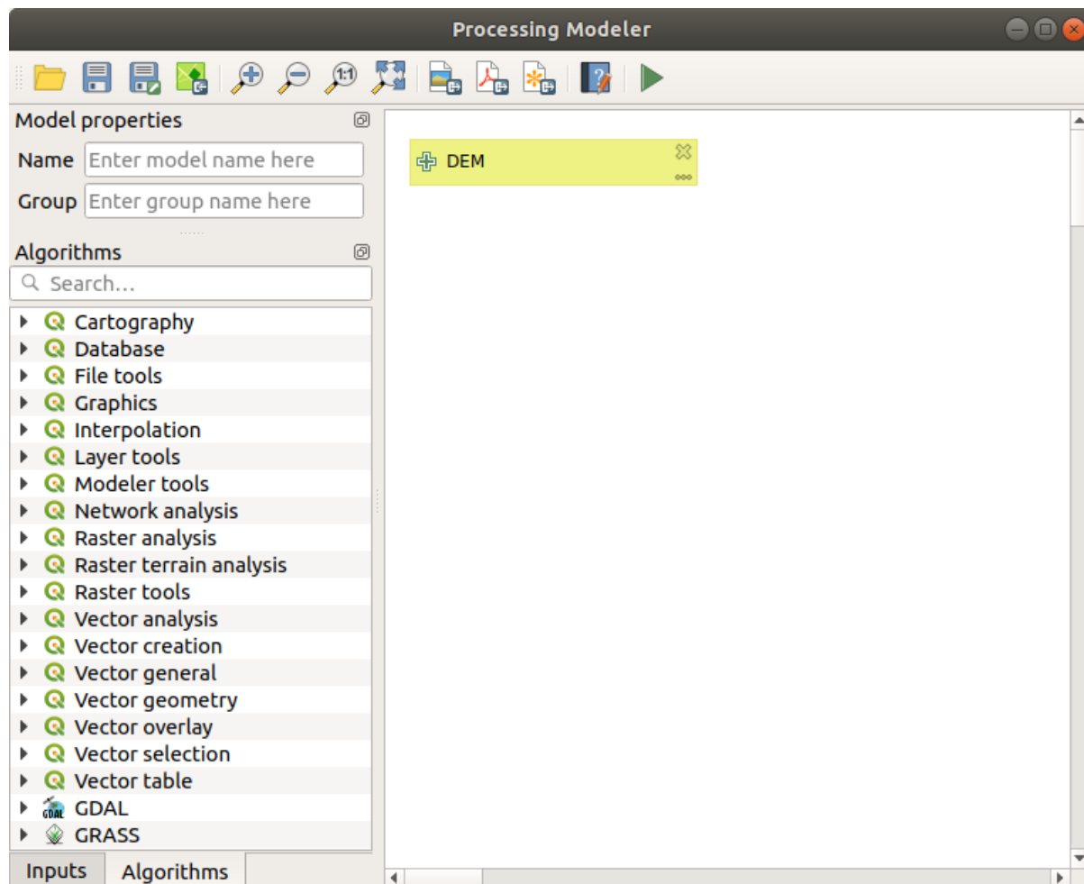
Рис. 21.21: Model Inputs
