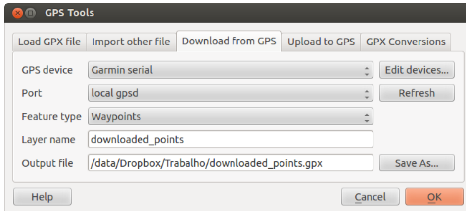
Рис. 18.2: Инструмент загрузки
