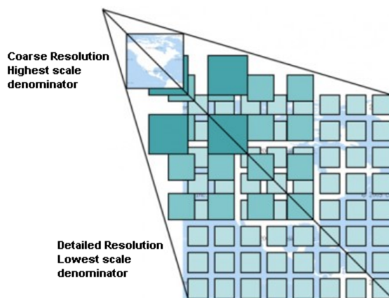
Figure 17.1: WMTS tiilijoukkojen konsepti
