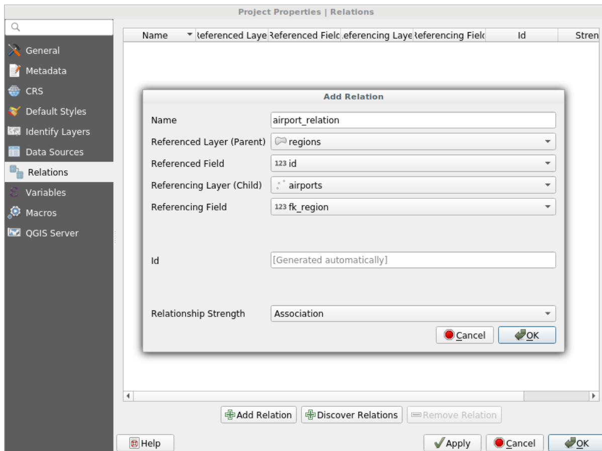
Figure 13.85: Administrador de relaciones
