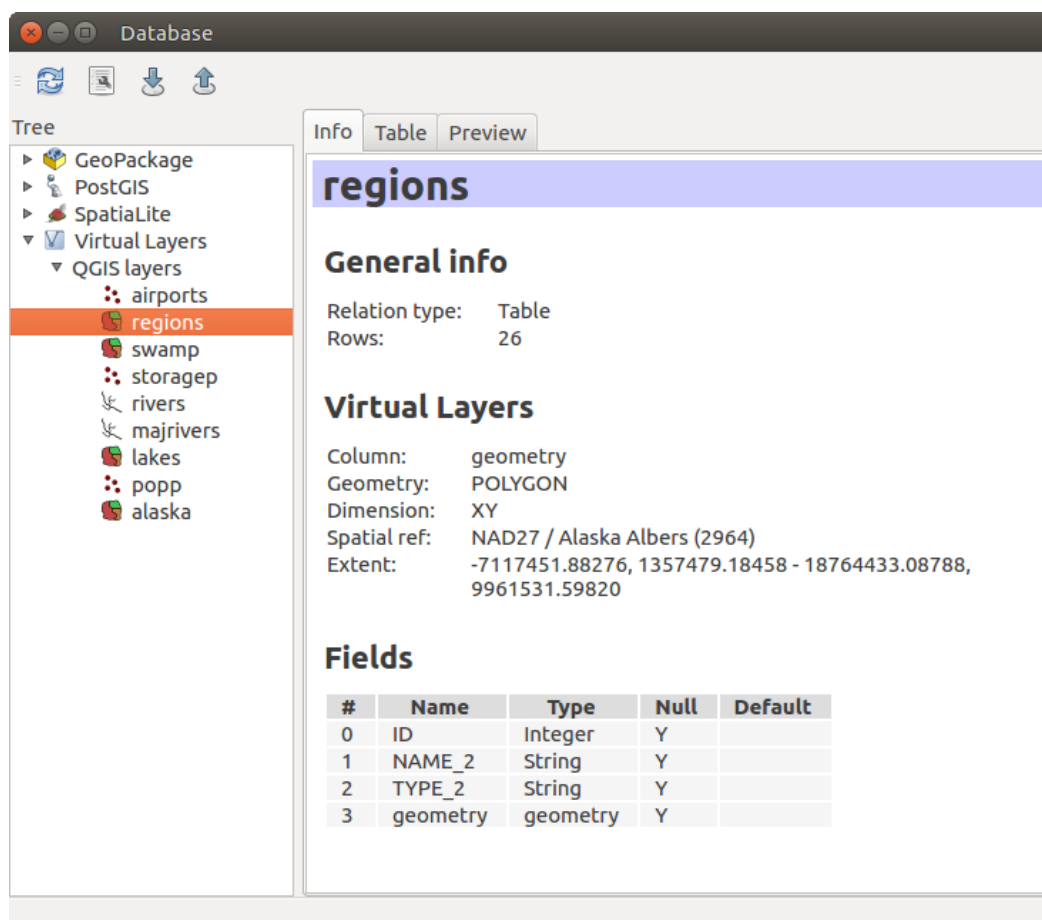
Figure 12.3: Diálogo del complemento administrador de BBDD
