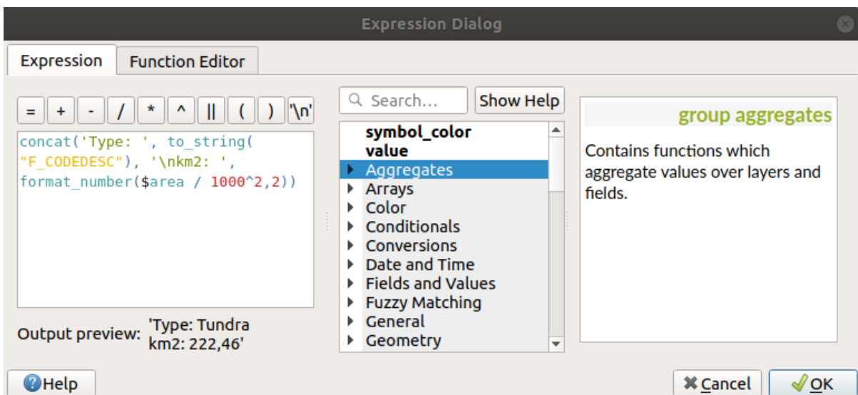
Figure 13.39: Usar expresiones para etiquetado
