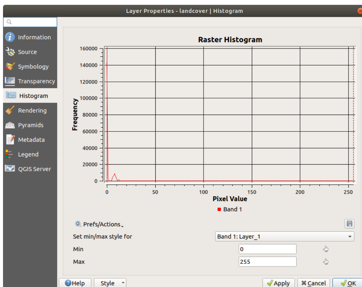
Figure 14.10: Histograma de Ráster
