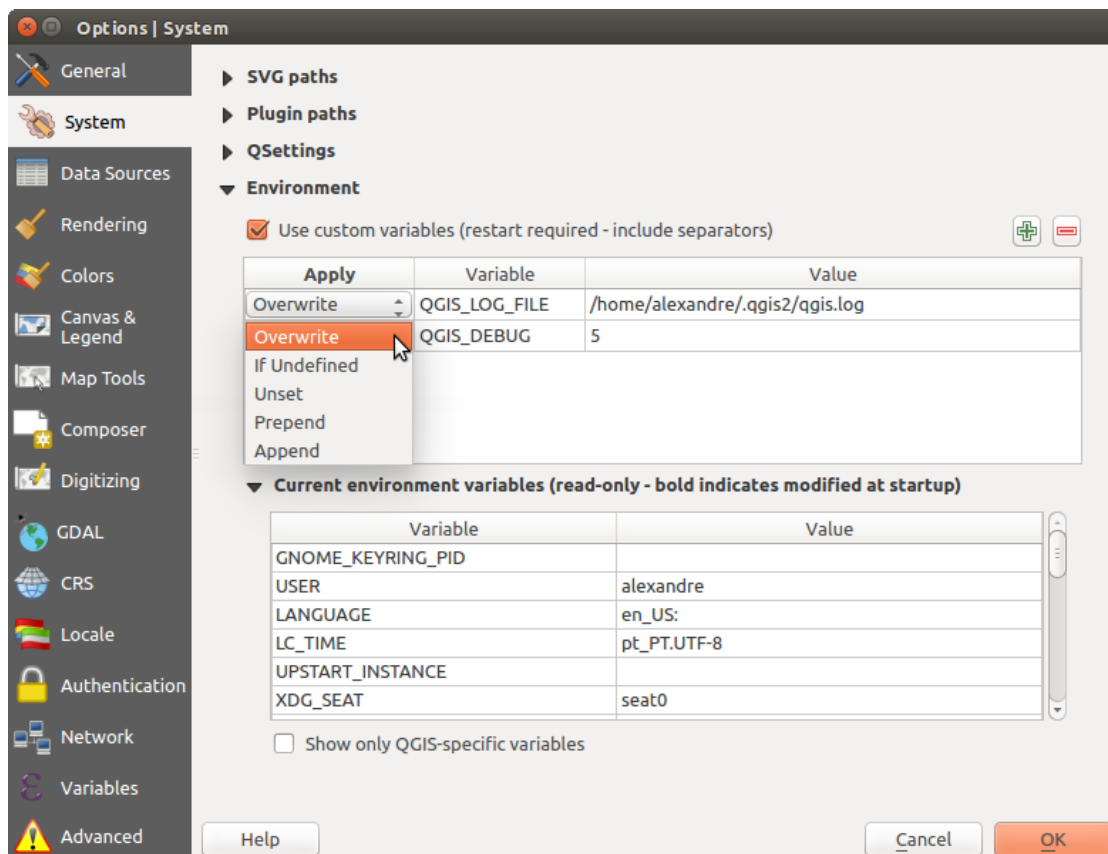
Figure 9.1: Variables del ambiente del sistema en QGIS
