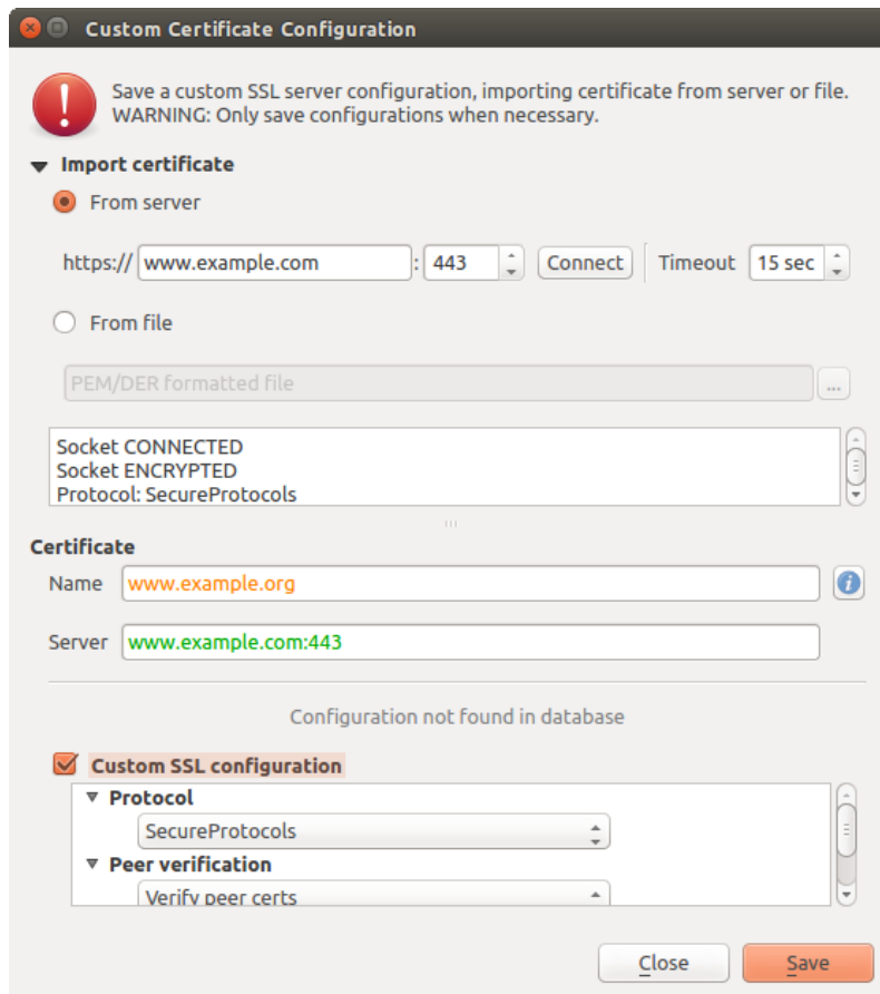
Figure 19.36: Adición manual de configuración
