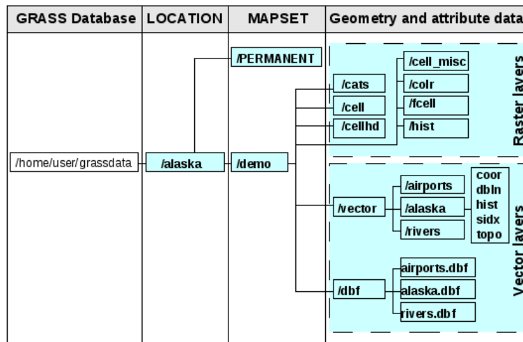
Figure 20.1: Datos GRASS en la LOCALIZACIÓN alaska
