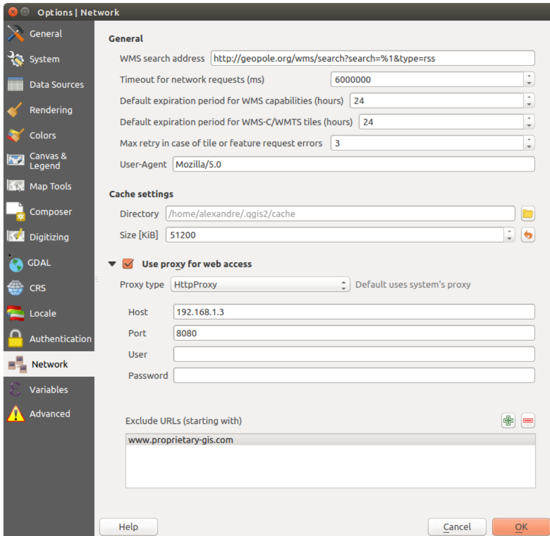
Figure 9.15: Configurar proxy en QGIS
