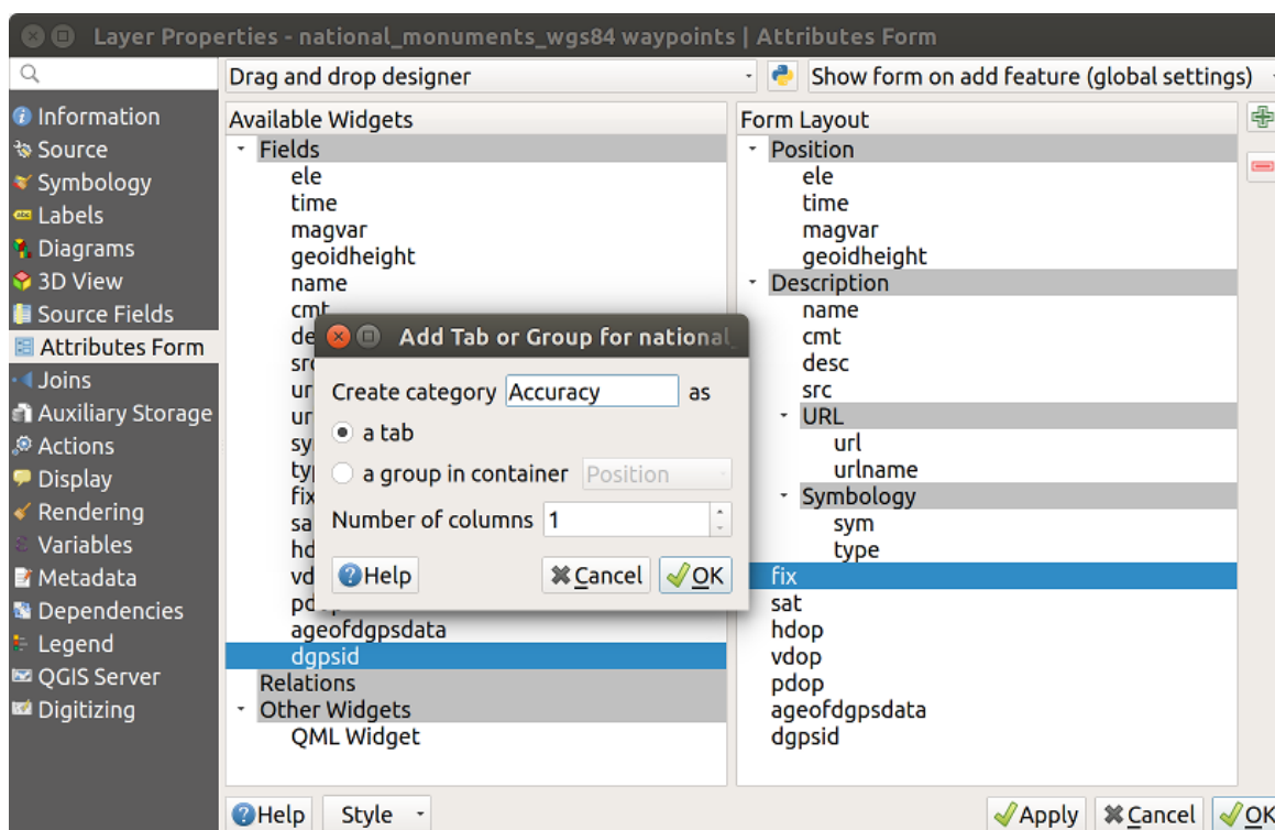
Figure 13.51: El cuadro de diálogo para crear categorías con el Diseño del editor de atributos
