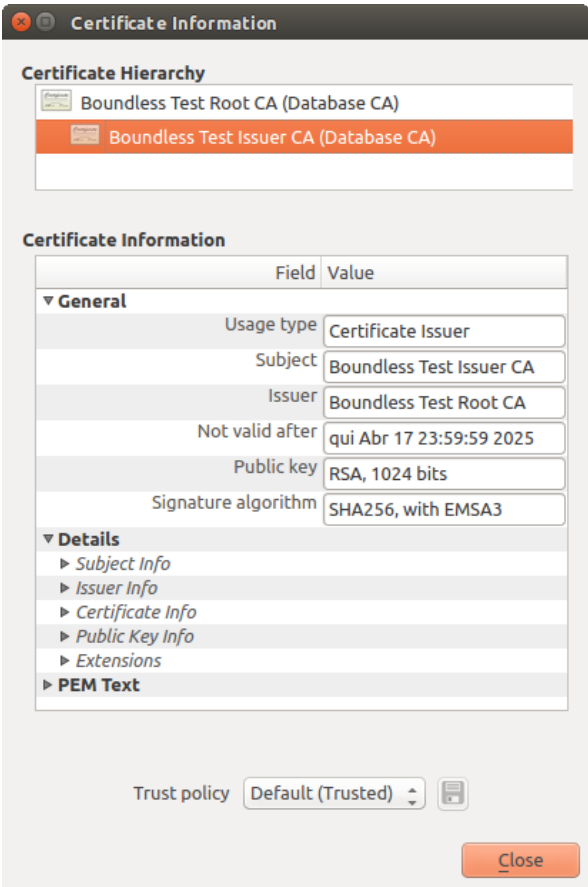
Figure 19.25: Dialogo de Información del certificado
