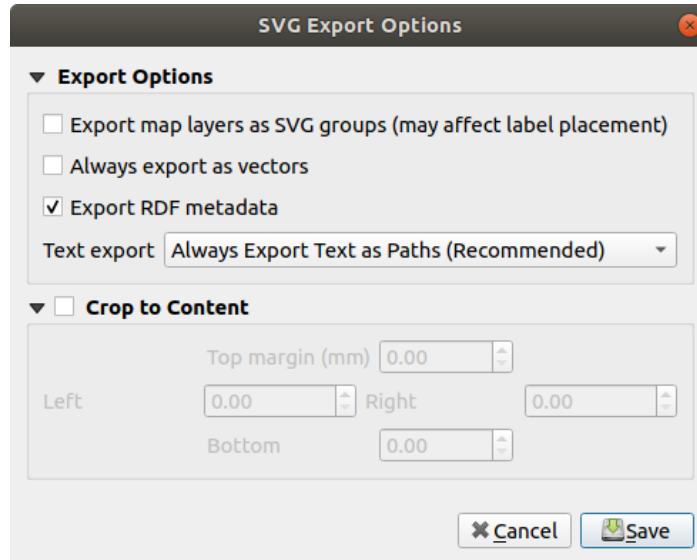
Figure 16.55: Opciones de Exportación de SVG
