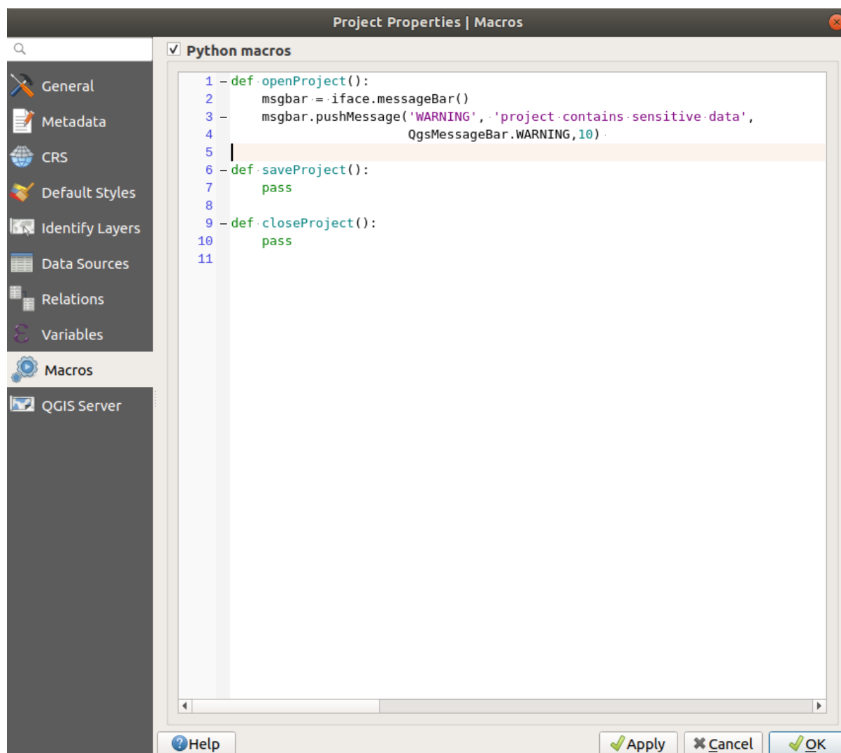
Figure 9.21: Definición macro en QGIS
