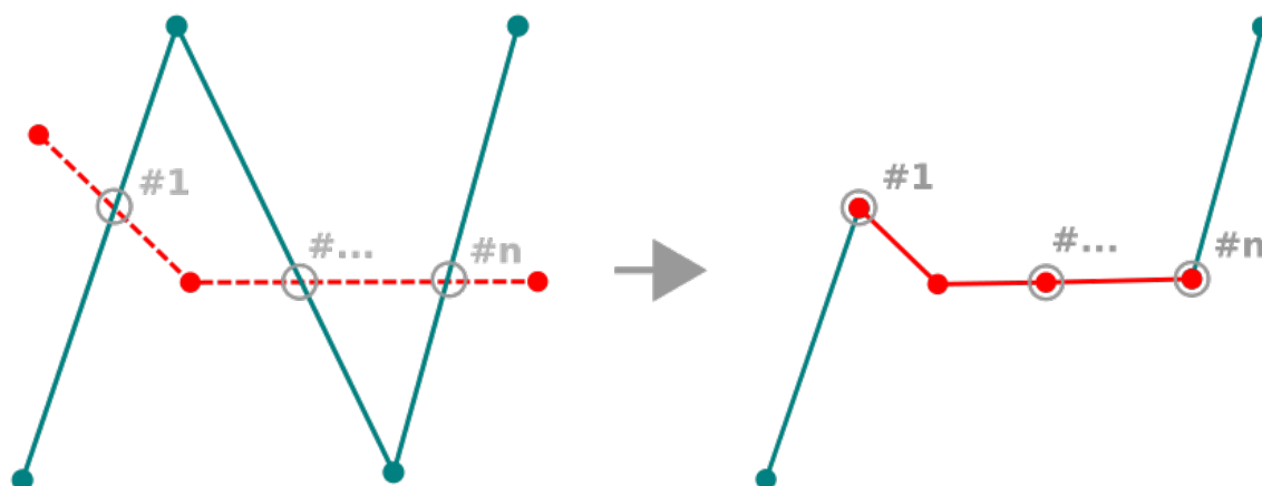
Figure 13.98: Remodelar línea
