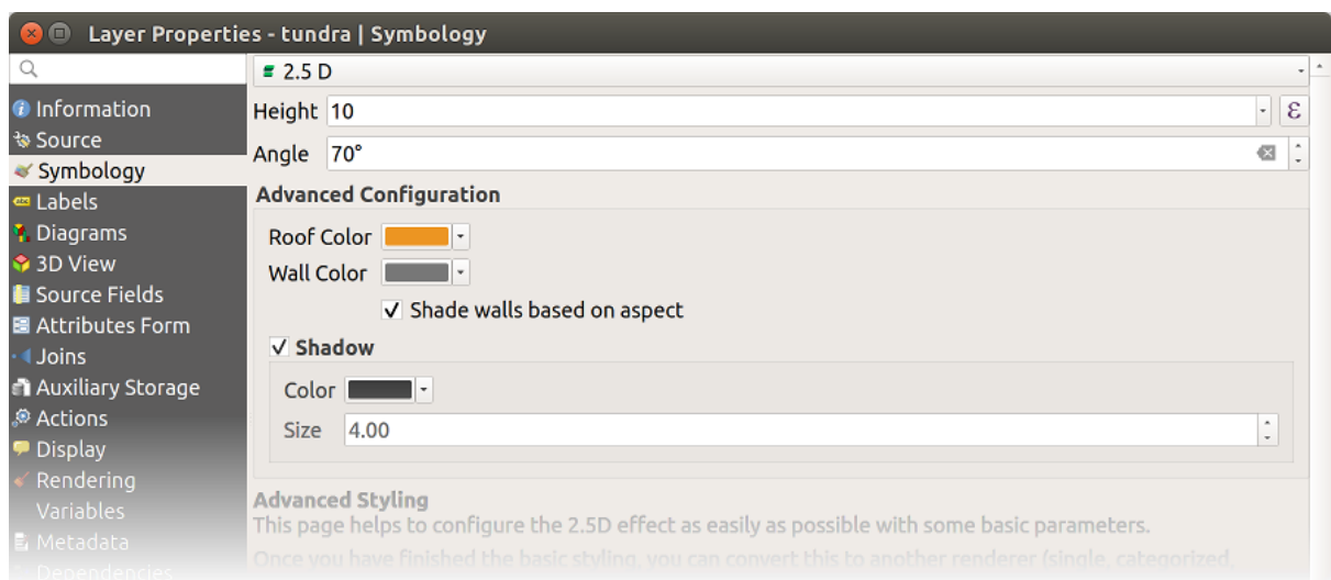
Figure 13.20: Diálogo 2.5D
