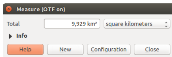
Figure 11.15: Medir Área
