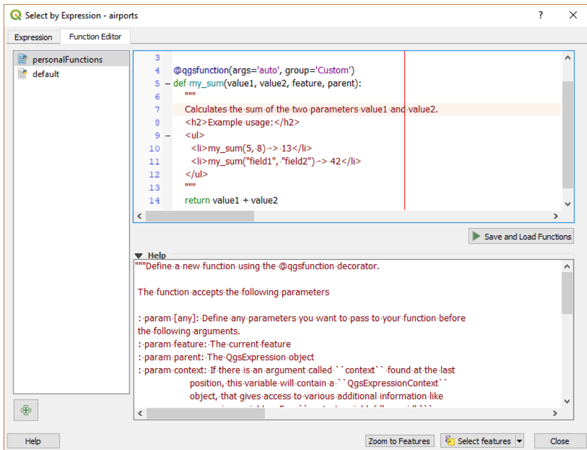
Figure 13.74: La pestaña Editor de funciones
