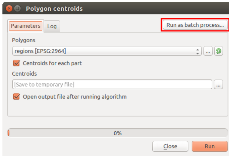
Figure 21.29: diálogo de procesamiento por lotes de algoritmo
