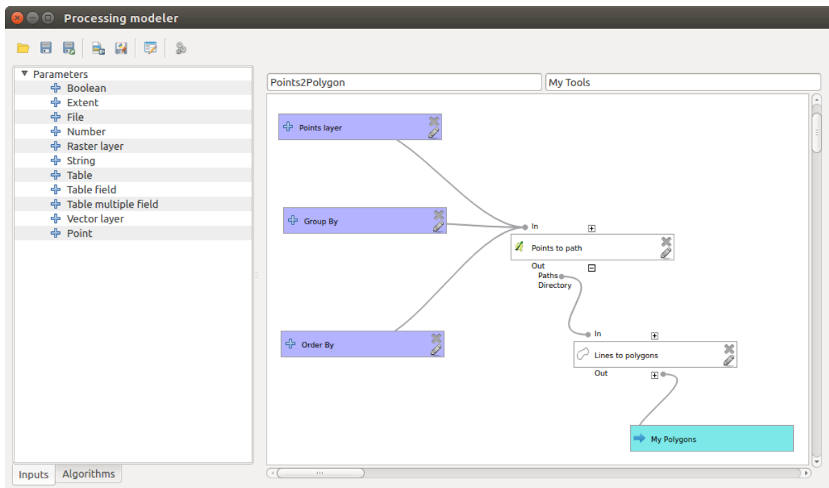
Figure 21.2: Procesamiento del modelador
