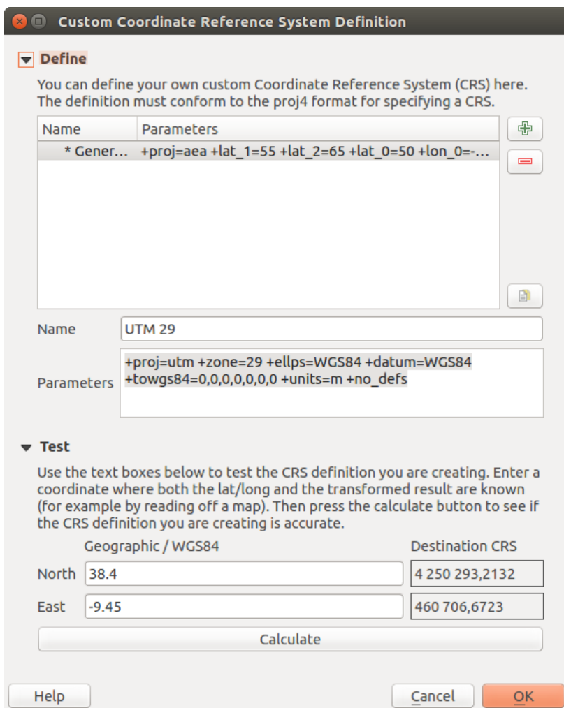
Figure 10.3: Dialog vlastní CRS
