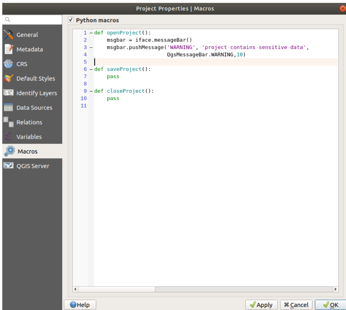
Figure 9.21: Makro nastavení v QGIS
