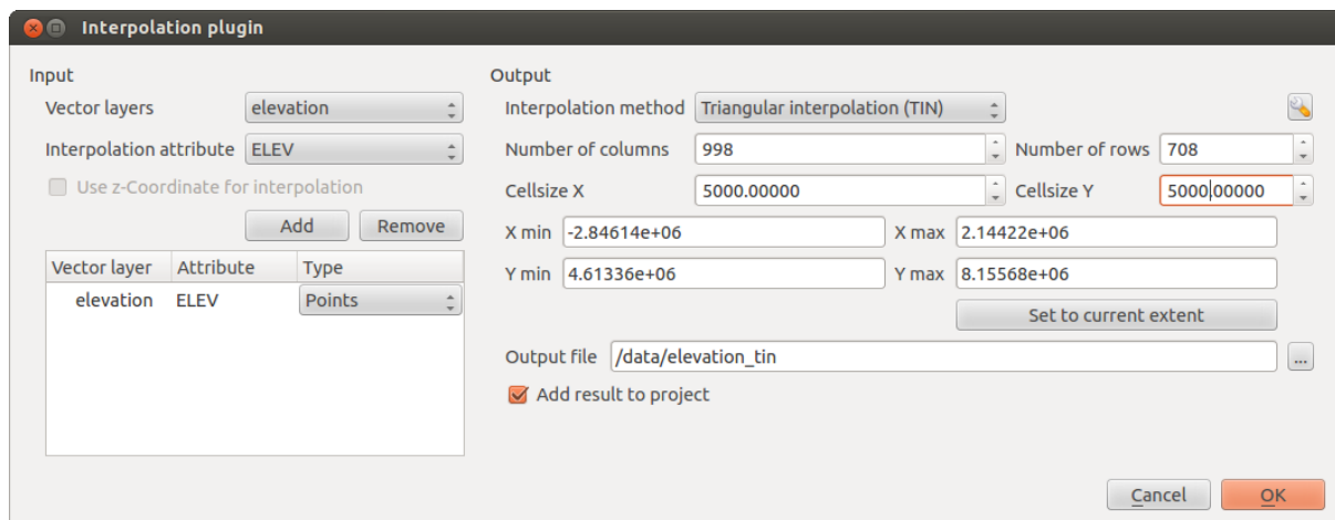
Gambar 20.27: Plugin Interpolasi
